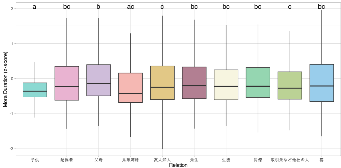
図 2 発話の向け先ごとの発話の平均モーラ長の分布。グラフの上に付した文字が TukeyHSD 検定 ( p < 0.05 ) によるグループを表しており、同じ文字であれば有意差がないことを意味する
